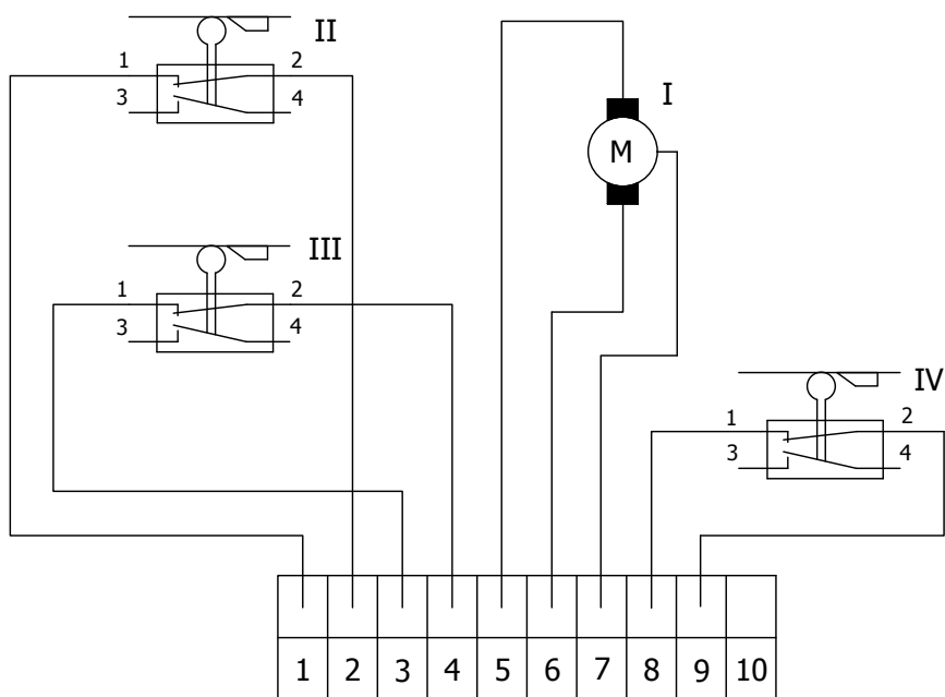
Schemat połączeń NS-EL 30
