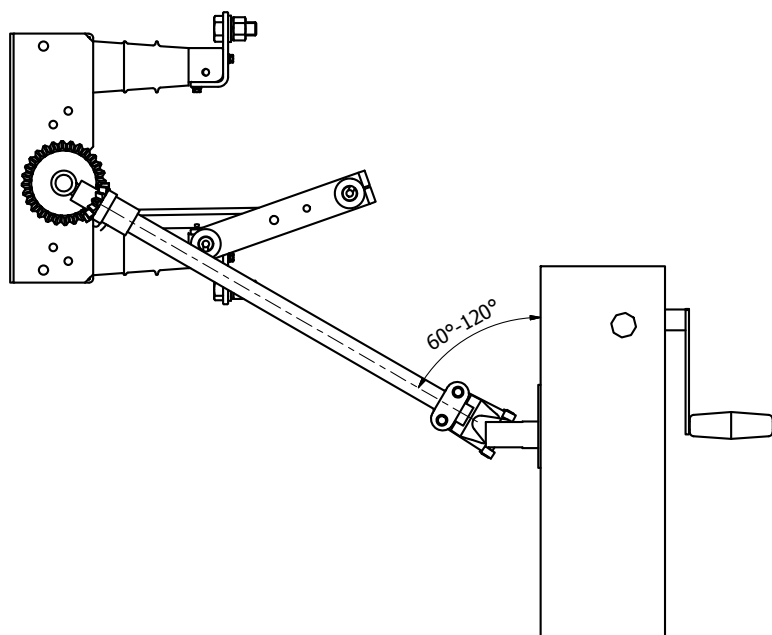
Podłączenie napędu do odłącznika
